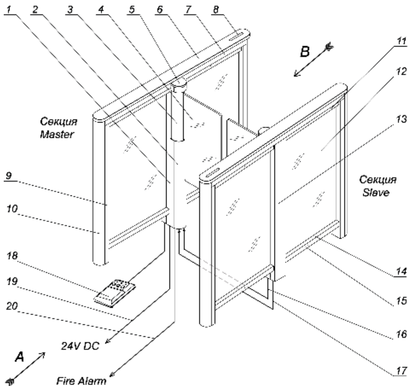
Рисунок 6. Внешний вид и устройство PERCo-ST-11:
