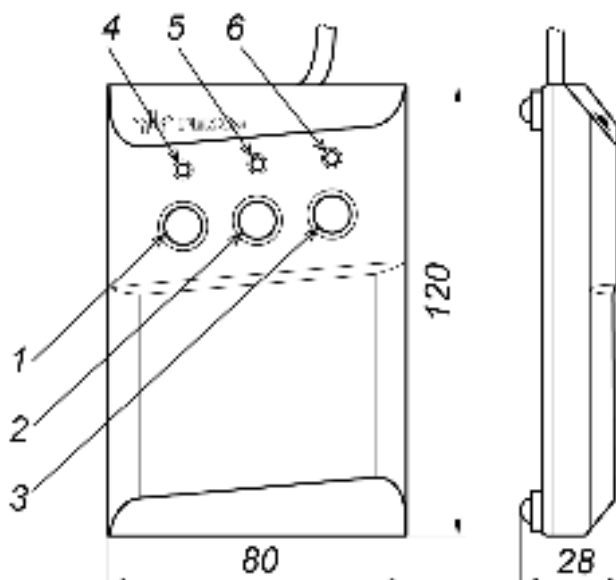
Рисунок 8. Общий вид и габаритные размеры ПДУ:
