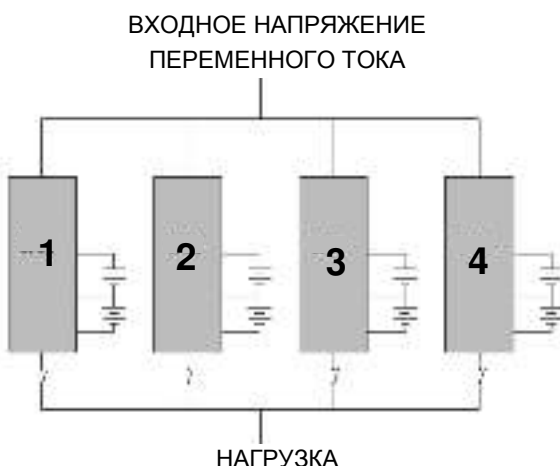
Рисунок 24 — Схема подключения изделий в систему параллельного резервирования.
