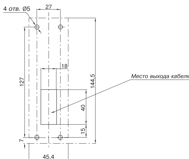
Разметка отверстий для установки считывателя
