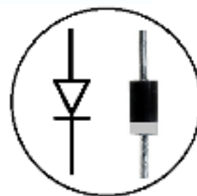
Маркировка диода 1N4004
