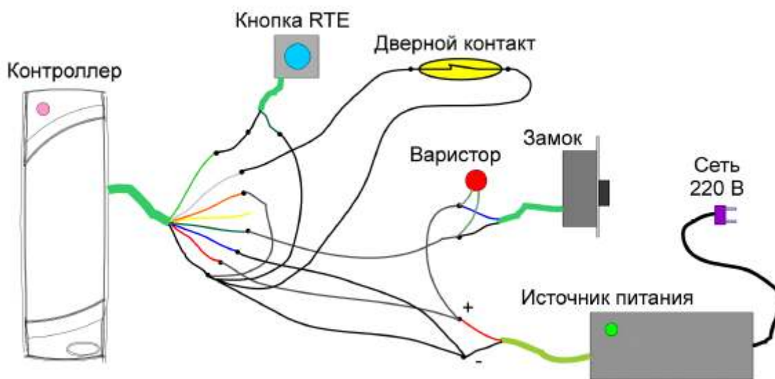
Рисунок 2. Схема подключения контроллера.
