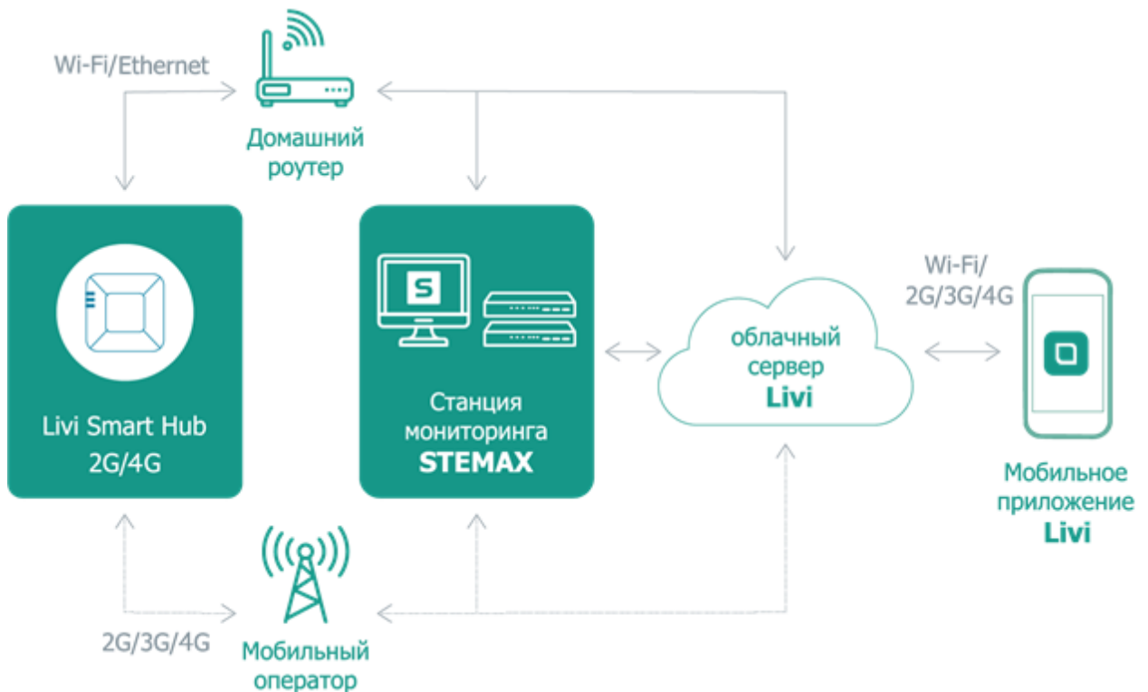
Рисунок 1.1 – Схема передачи извещений хабом
