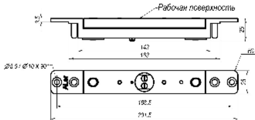
Рис.4 Якорная часть.
