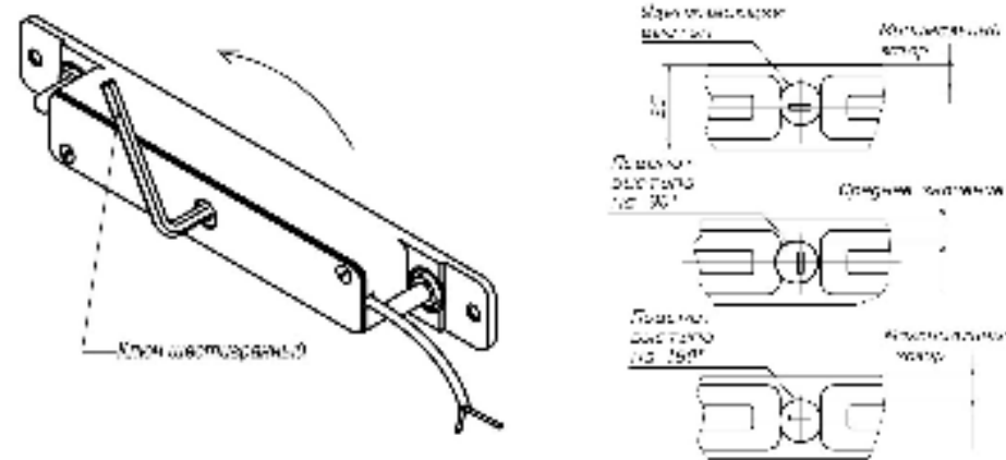
Рис. 8 Эксцентриковая регулировка зазора.
