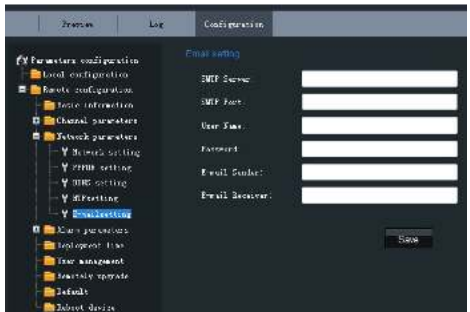
Рисунок 2.1.21: Настройки E-mail.
