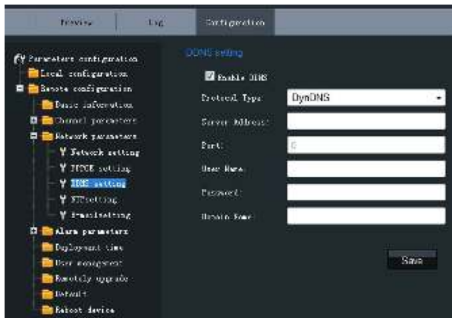
Рисунок 2.1.17: Настройки DDNS.
