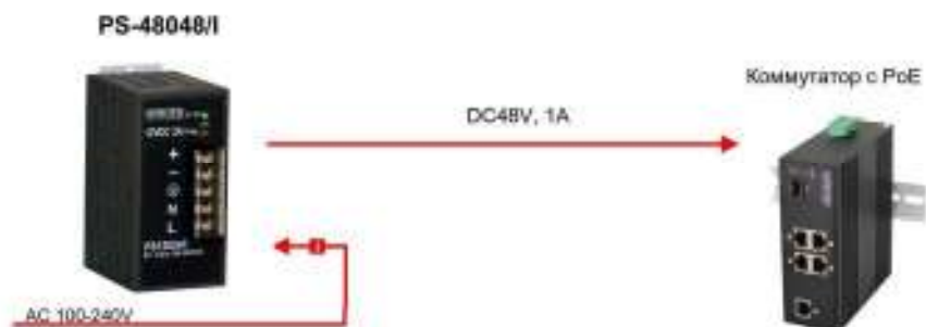
Рис. 5 Подключение PS-48048/I
