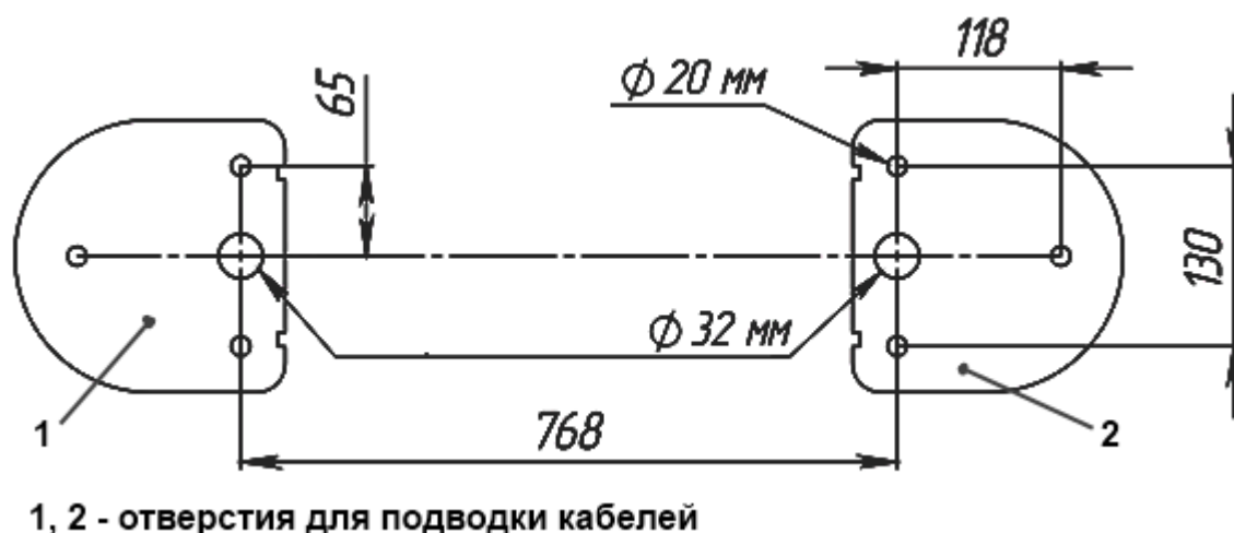
Рисунок 4 – Установочные размеры площадки турникета
