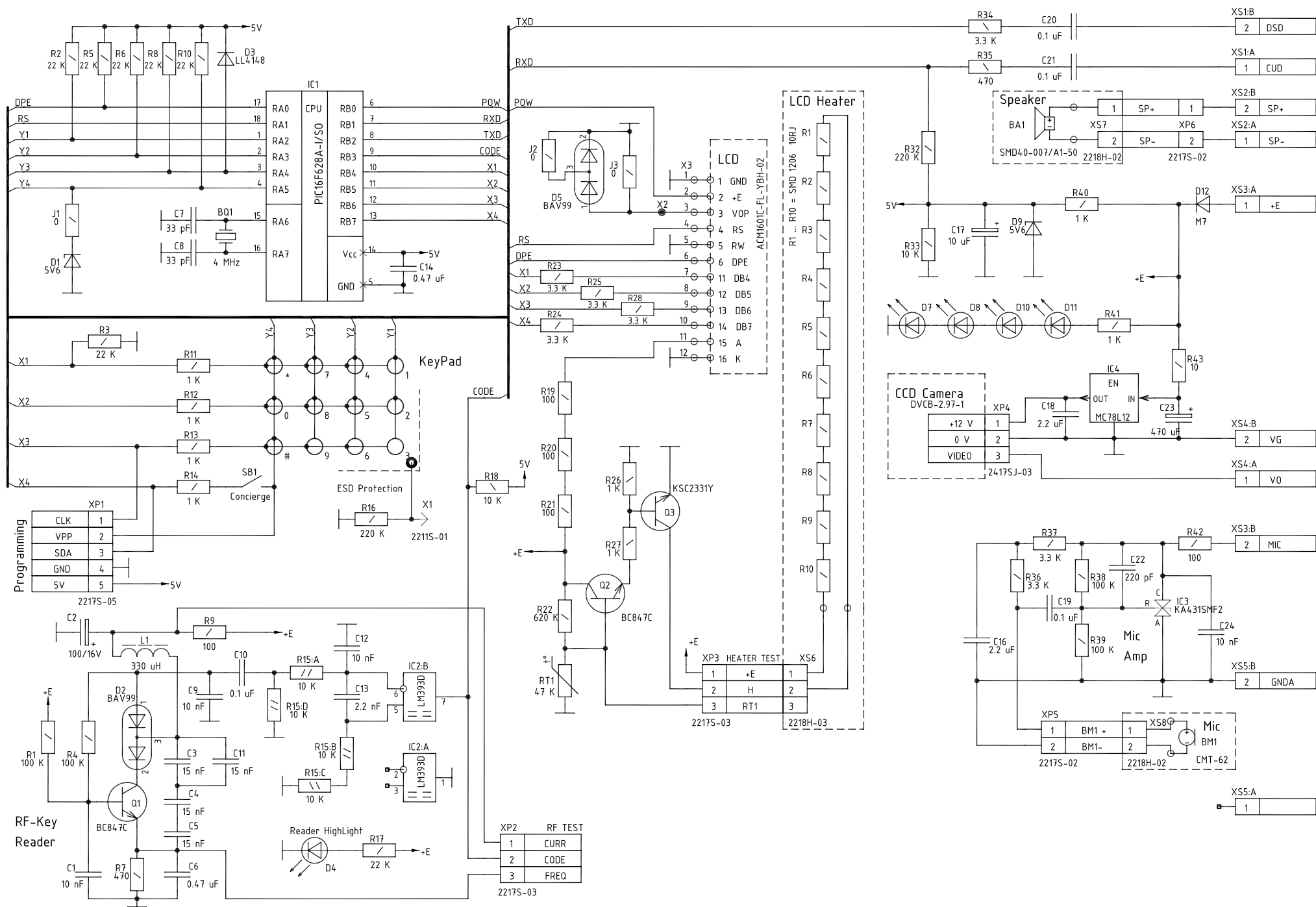
Блок вызова БВД-432 RCB Схема электрическая принципиальная
