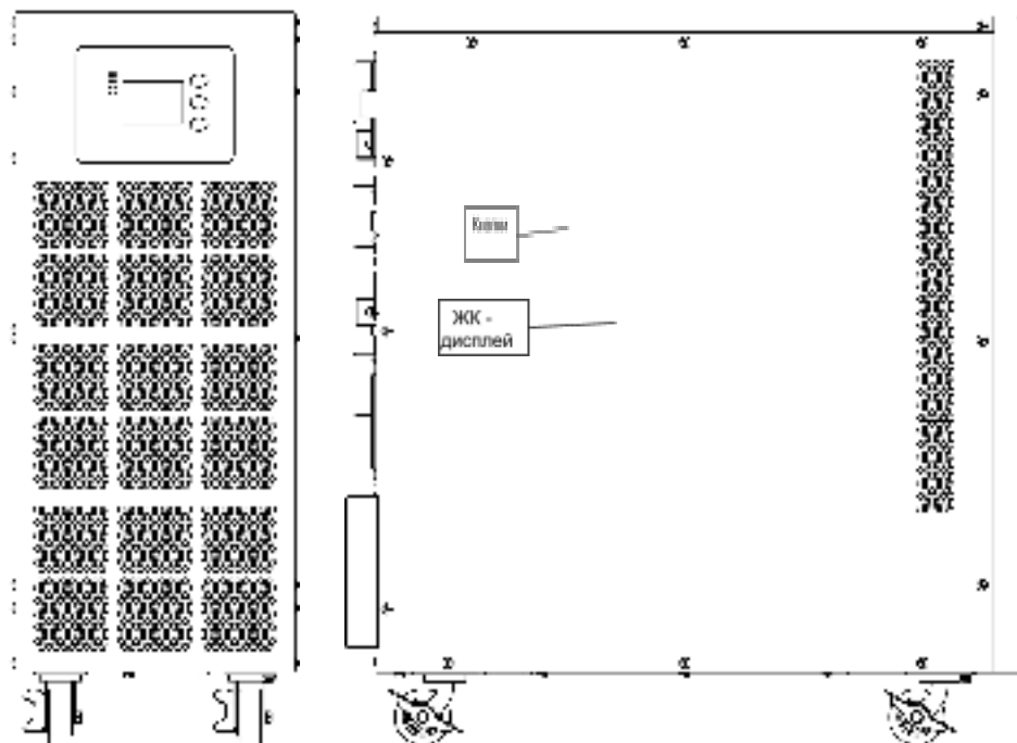
Рисунок 1 - Общий вид изделия спереди и слева
