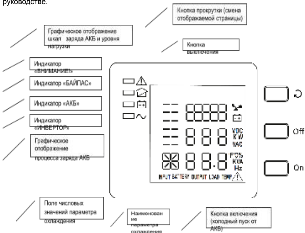
Рисунок 3 - ЖК—дисплей
