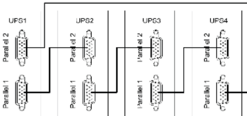
Рисунок 25 — Схема соединения изделий в «кольцо» через параллельные порты.
