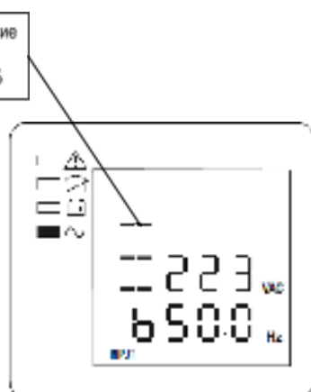
Рисунок 22 — ЖК-дисплей, плавающий (поддерживающий) заряд АКБ
