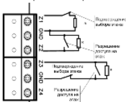
Рис.6. Примеры подключения шлейфов
