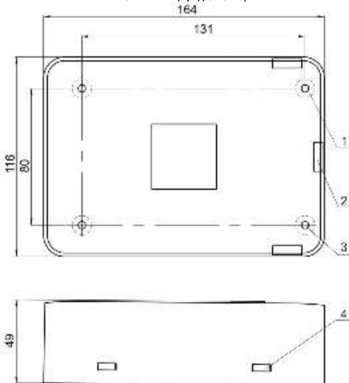
Рисунок А2. Габаритные и установочные размеры прибора ВЗРС-ПК1(ТМ)-01 Версия 3.2.
