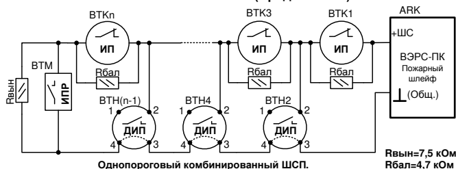
Рисунок.Б5. Комбинированная схема однопорогового ШСП.
