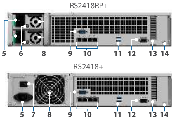
Задняя панель
