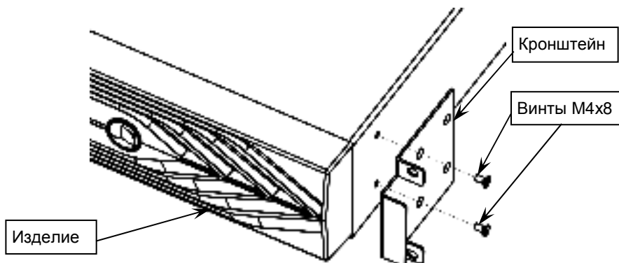
Рисунок 4 — Установка кронштейнов на корпус изделия
