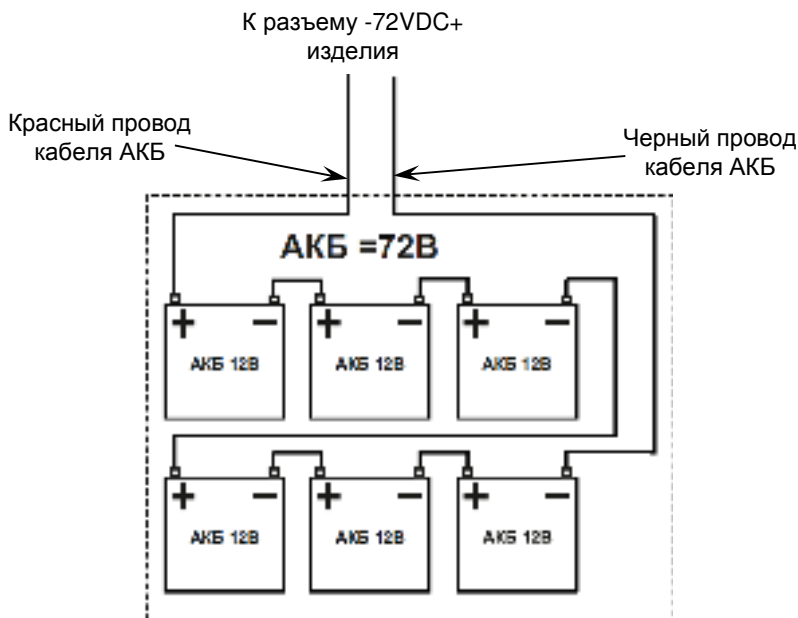
Рисунок 5 — Схема монтажа аккумуляторной батареи.
