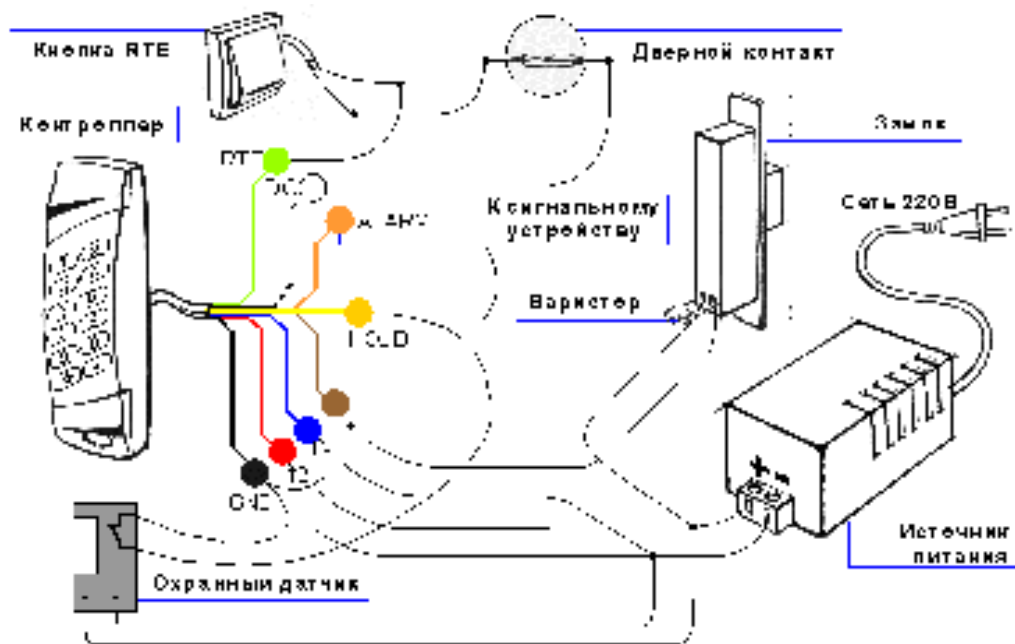
Рисунок 3. Подключение охранного датчика.
