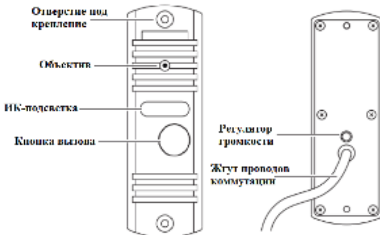
Рисунок 1. Внешний вид
