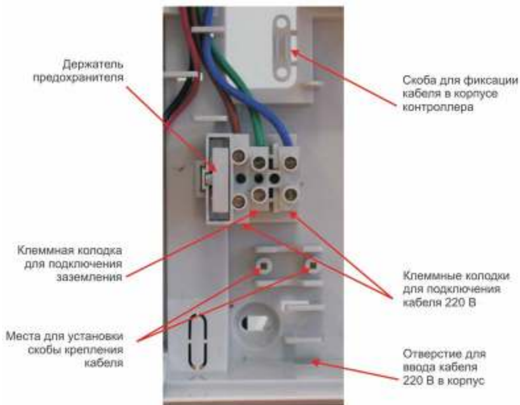
Рисунок 5. Подключение контроллера к сети 220 вольт.
