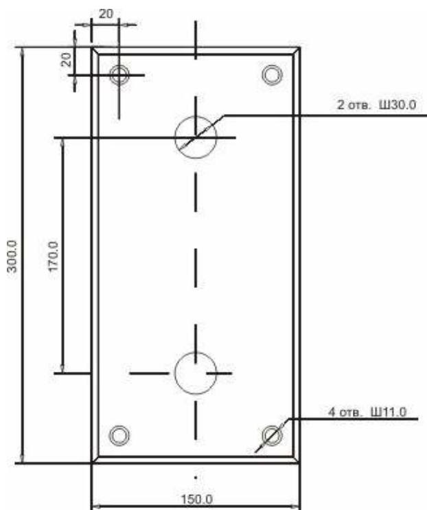
Рисунок 2. Габаритные размеры основания антенного модуля.
