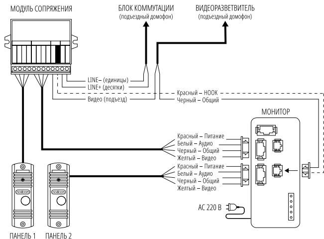
Рис. 15 Схема подключения монитора серии UNIT к подъездному домофону через модуль сопряжения
