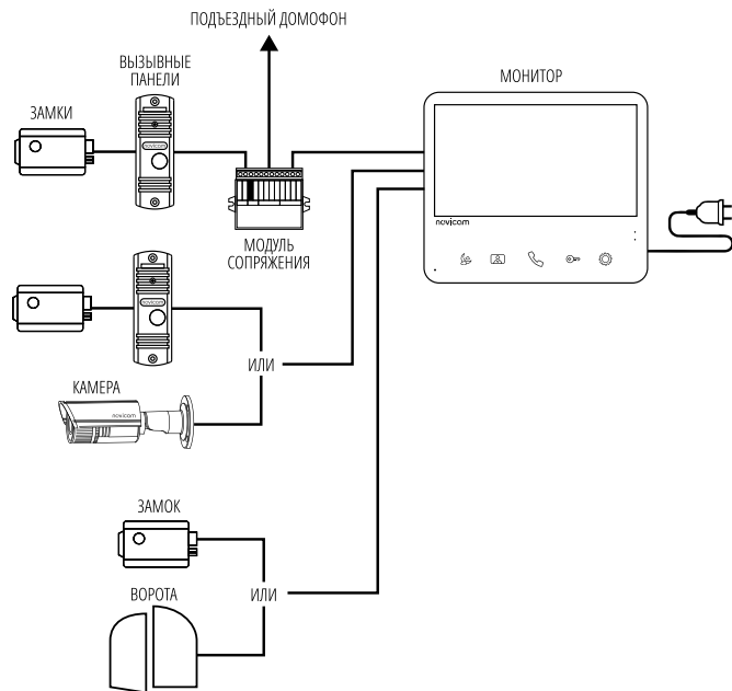
Рис. 13 Функциональная схема системы на базе видеодомофонов UNIT 4 | UNIT 7
