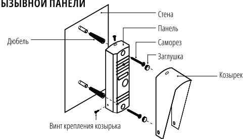
Рис. 7 Фронтальная установка вызывной панели
