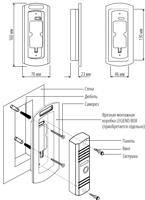
Рис. 9 Врезной монтаж вызывной панели
