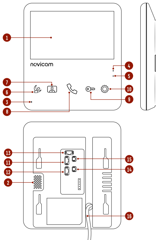
Рис. 2. Монитор видеодомофона UNIT 4
