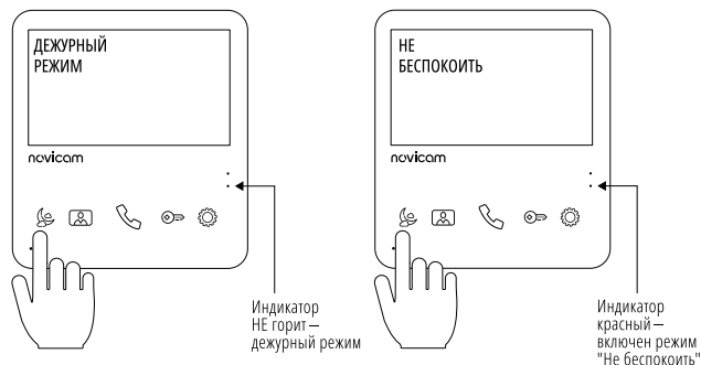
Рис. 18 Активация/деактивация режима "Не беспокоить"
