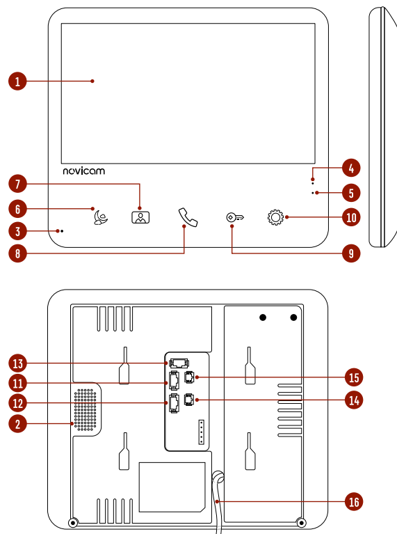
Рис. 3. Монитор видеодомофона UNIT 7
