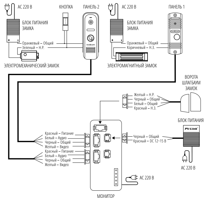
Рис. 14 Общая схема подключения видеодомофонов серии UNIT
