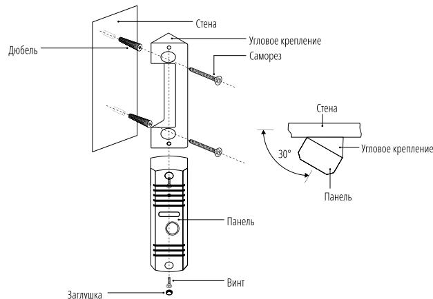
Рис. 8 Установка вызывной панели под углом 30°
