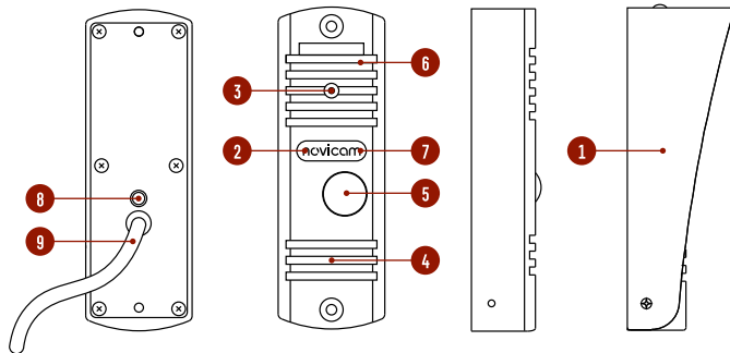
Рис. 4 Вызывная панель, входящая в комплекты UNIT 4 | 7 KIT
