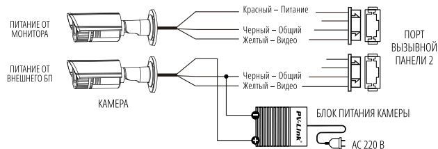
Рис. 16 Схема подключения видеокамеры к монитору UNIT
