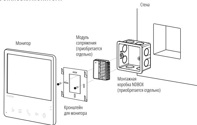
Рис. 6 Монтаж монитора UNIT
