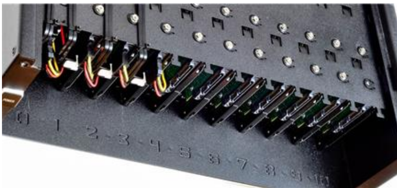
Рисунок 4. Дисковый отсек
