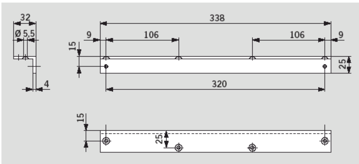
Монтажный уголок
