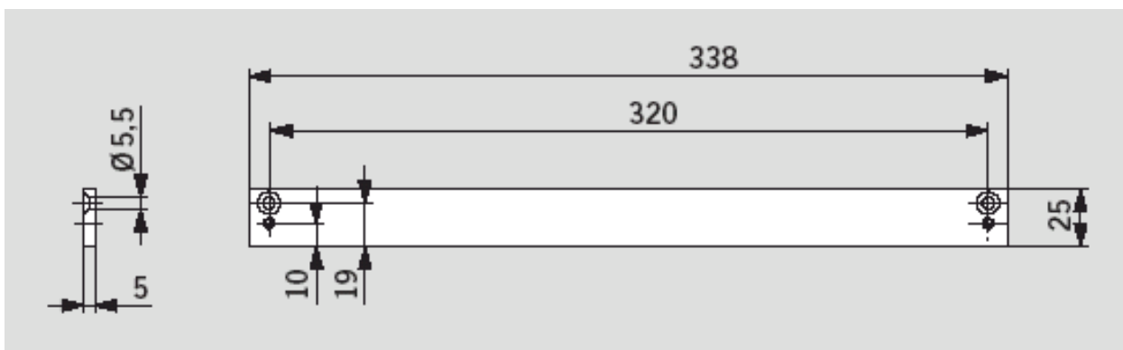
Монтажная пластина
