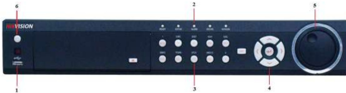
Рис. 3. Передняя панель цифрового регистратора
