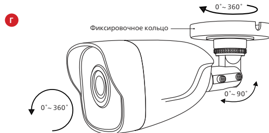
Рис. 12 Установка камеры NC33WP/NC43WP (шаг Г).
