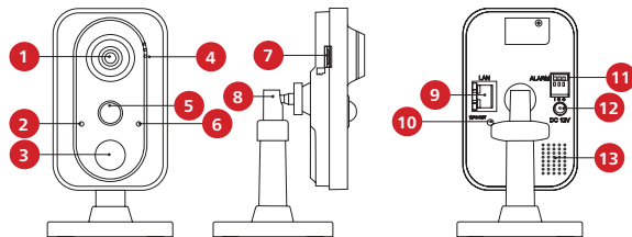
Рис. 5 Описание камер NC24FP/NC44FP.
