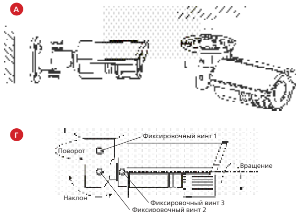
Рис. 18 Установка камеры NC39WP, NC49WP (шаги А,Б,Г).
