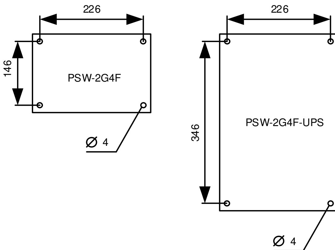
Рис. 6.1.1. Разметка крепления
