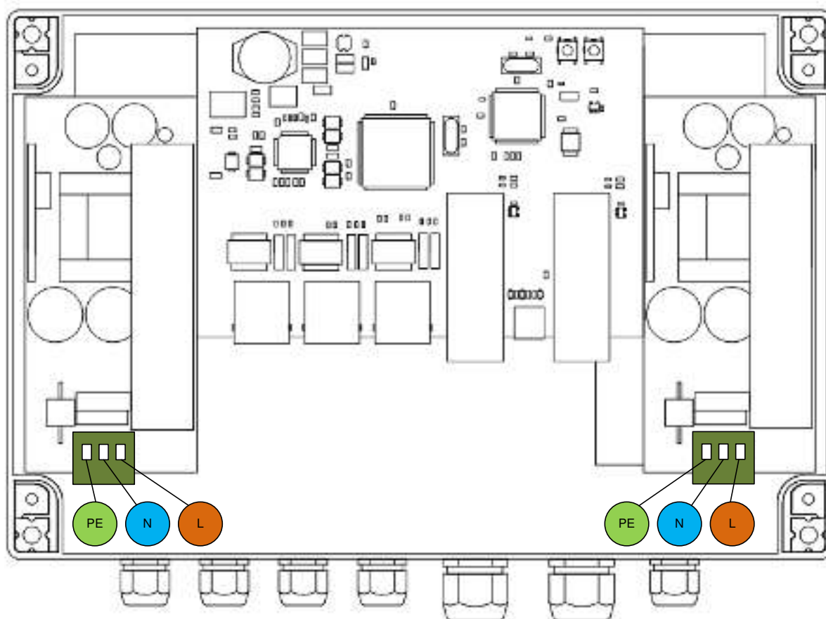
Рис. 6.3-1. Подключение питания к PSW-2G4F.
