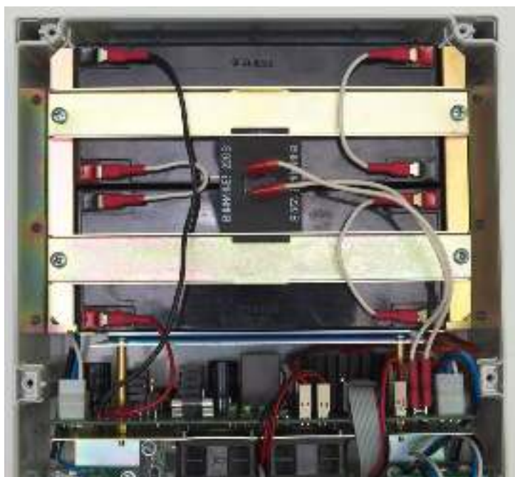
Рис. 2.9.5. Подключение АКБ.
