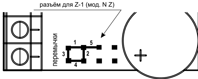
Рис. 3 Положение перемычек
