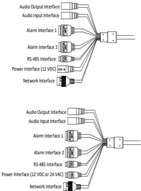
Рисунок 1-8 Описание кабелей
