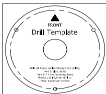
Рисунок 2-14 Шаблон крепления
