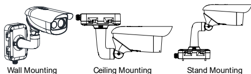
Рисунок 2-18 Методы установки камеры типа III
