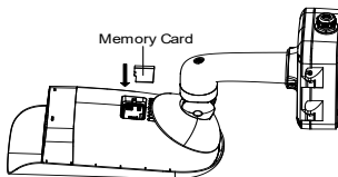
Рисунок 2-8 Установка карты памяти
