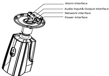
Рисунок 1-9 Описание интерфейсов
