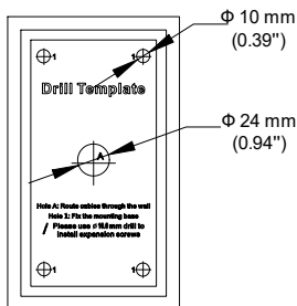
Рисунок 2-20 Шаблон крепления
