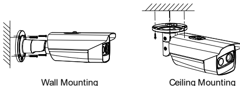
Рисунок 2-15 Установка на стену/потолок
