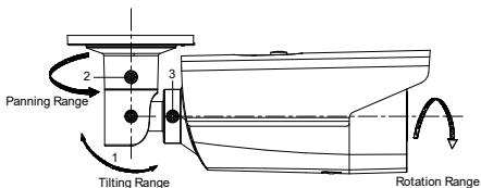
Рисунок 2-16 3-х осевая регулировка
