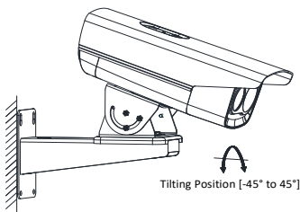
Рисунок 2-13 Регулировка наклона
