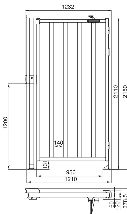
Габаритные размеры калитки
