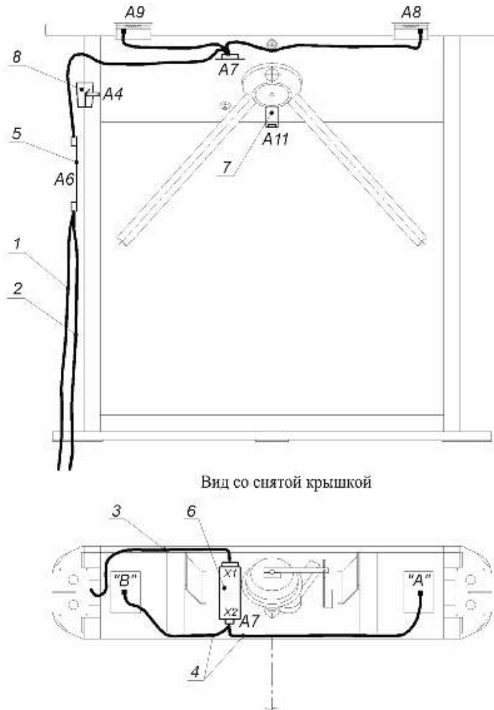
Рисунок 11. Схема прокладки кабелей в стойке турникета:
