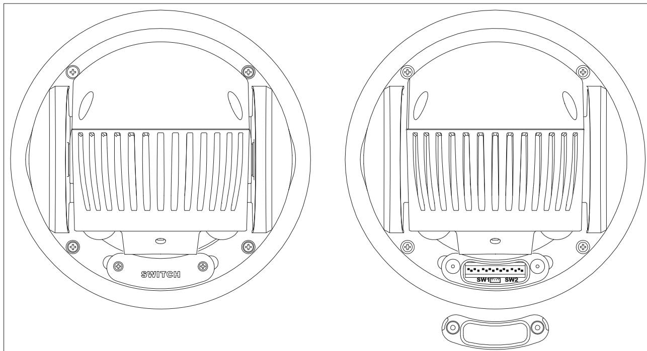
Рис. 1.3. Расположение DIP-переключателей
