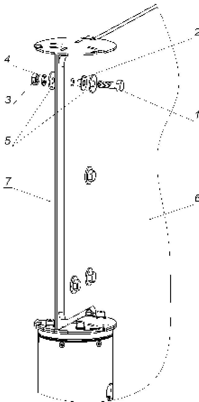
Рисунок 12. Установка створки
