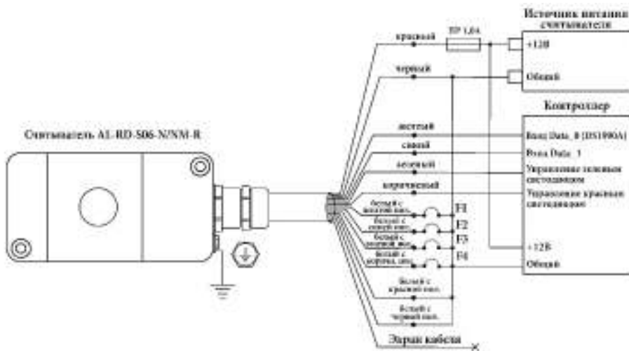
Рисунок 2 – Схема подключения счетчиков AL-RD-S06-N/NM-R- (-К, -М, -Т) с небронированным кабелем к контроллеру СКУД.
