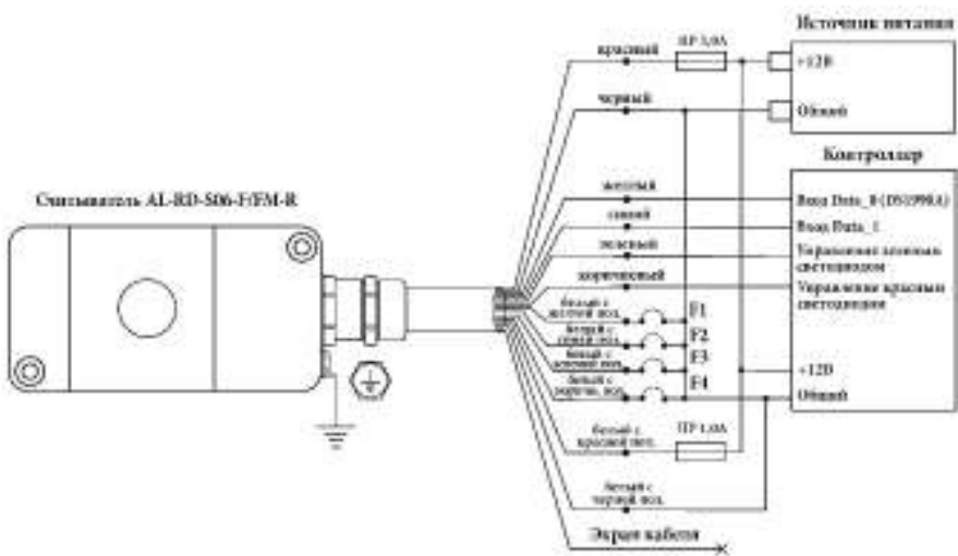
Рисунок 5 – Схема подключения счетчика AL-RD-S06-F/FM-R к контроллеру СКУД с питанием счетчика и нагревателя от одного источника питания.
