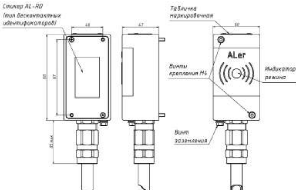
Рисунок 1 - Габаритно-установочные размеры считывателя AL-RD-S06-F/N-R
