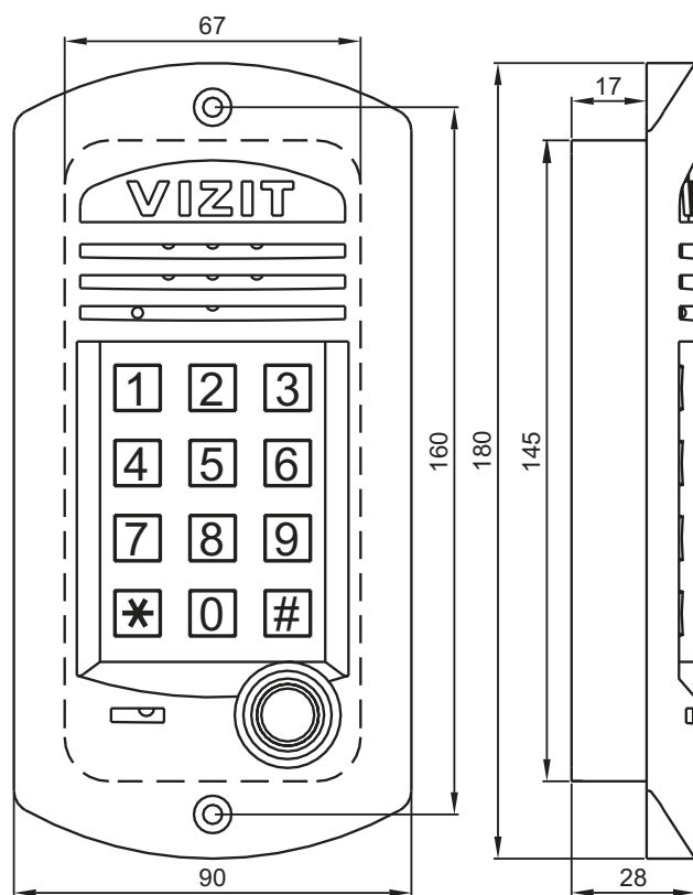
Рисунок 4 - Габаритные и установочные размеры блока вызова
