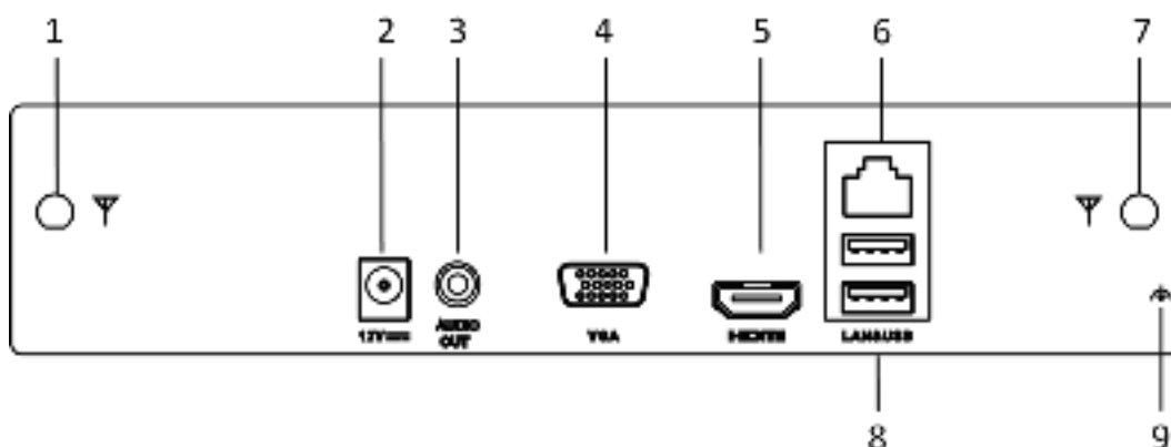
Рисунок 1-2 Задняя панель
