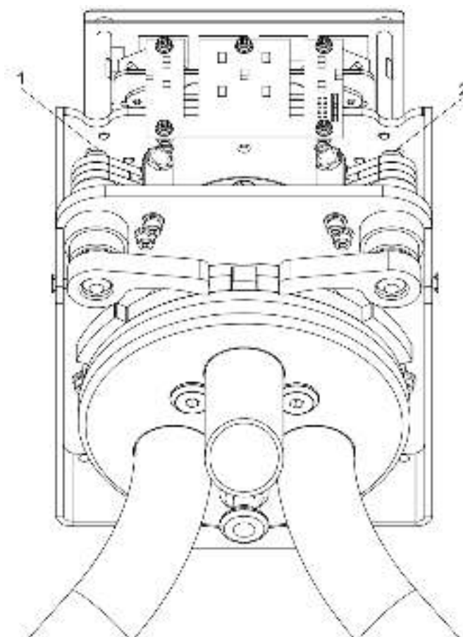
Рисунок 12 – Элементы механизма турникета
