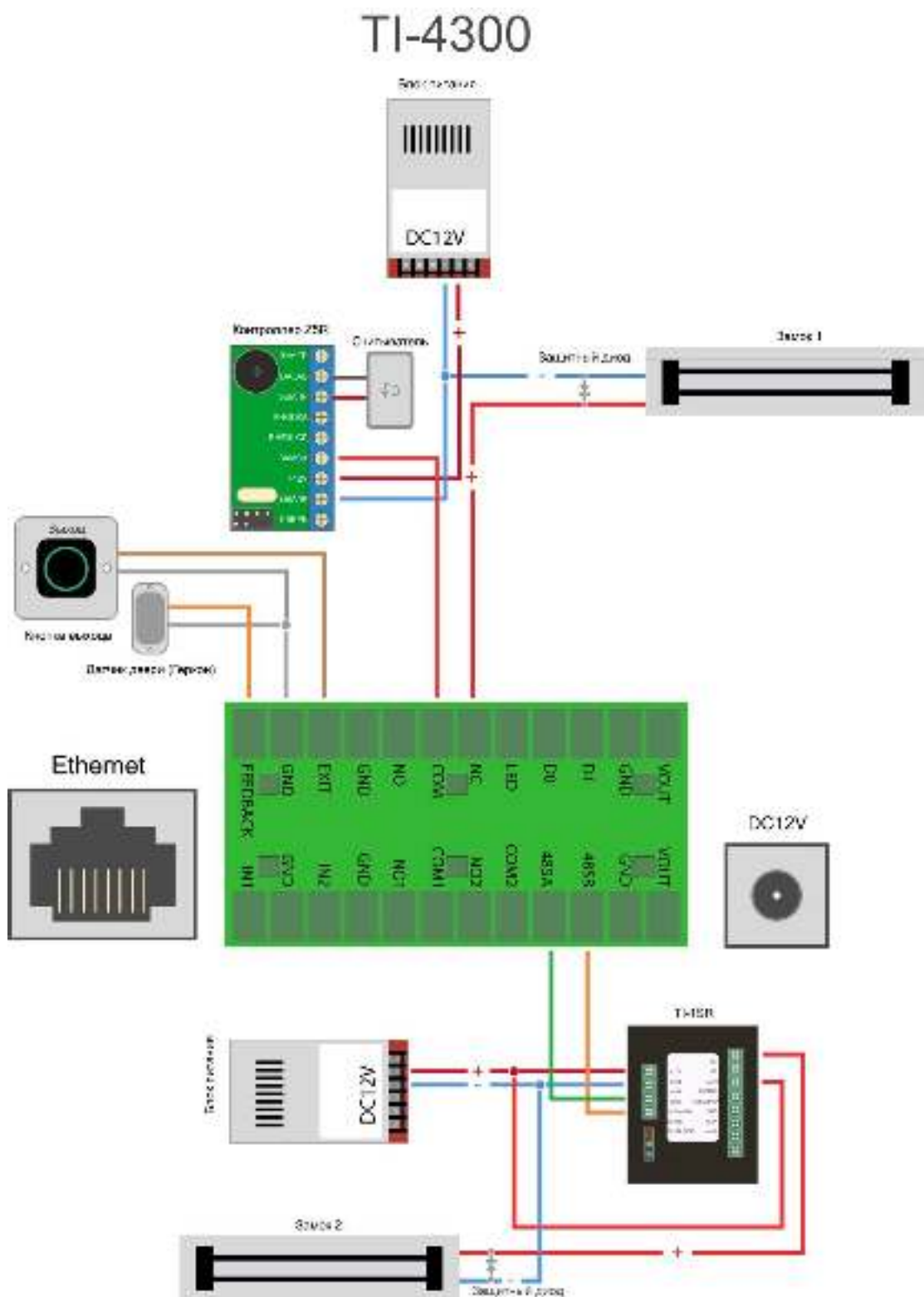
Схема подключения дверного замка и кнопки выхода:
