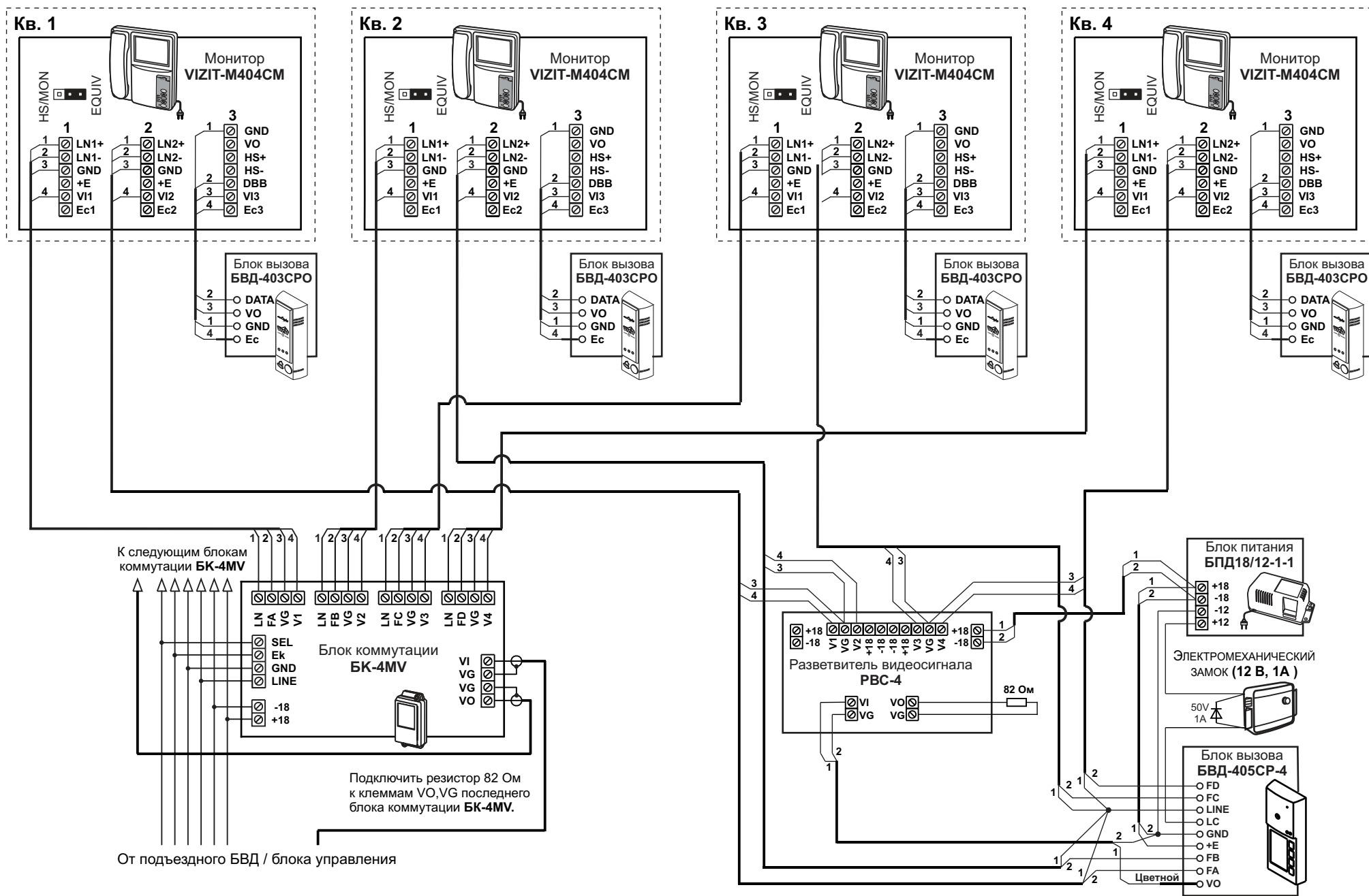
Рисунок 8 - Схема соединений монитора VIZIT-M404CM с блоком коммутации БК-4MV и блоком вызова БВД-405СР-4
