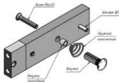
Рисунок 2 - Комплект крепления якоря
