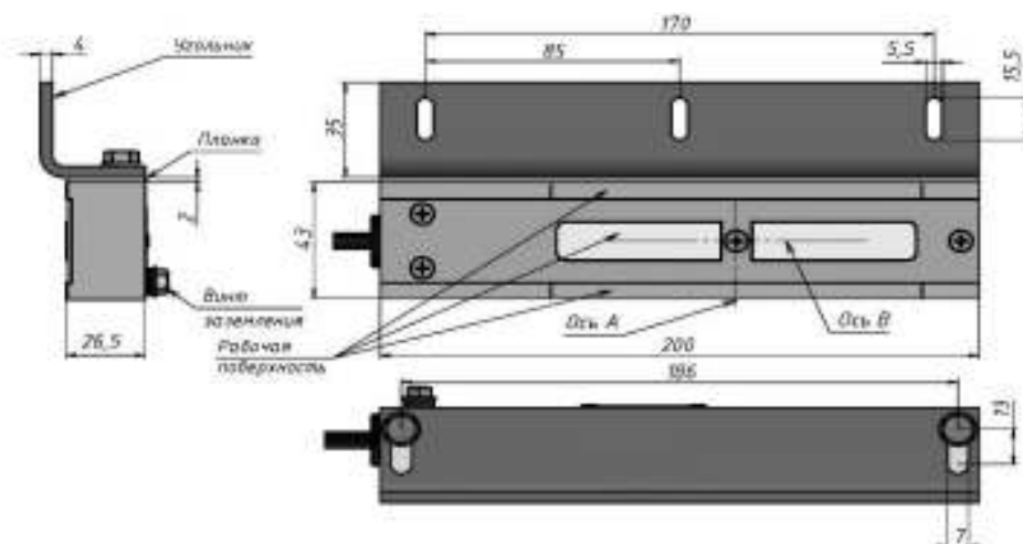
Рисунок 4 - Корпусная часть
