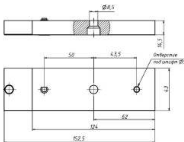
Рисунок 5- Габаритный чертеж якоря
