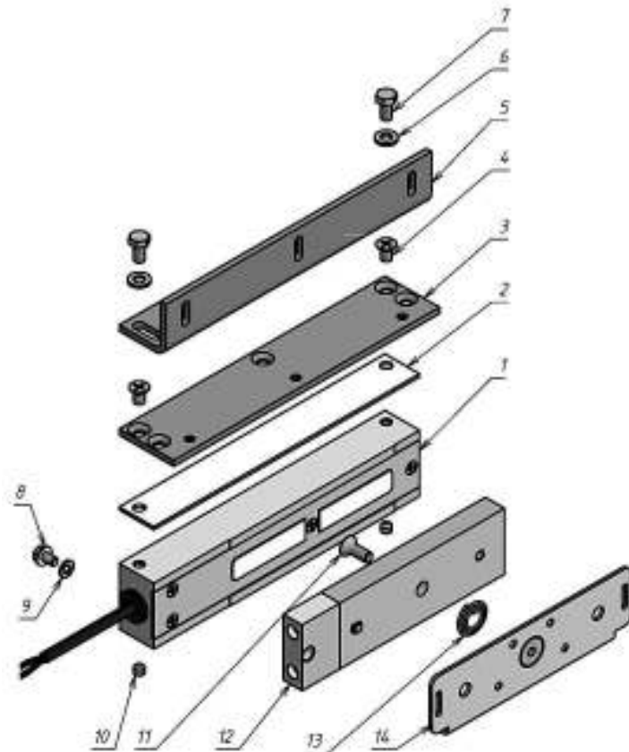
Рисунок 1 – Комплект поставки
