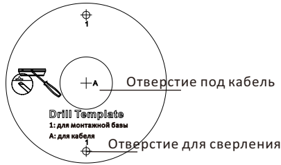
Рисунок 2-2 Шаблон крепления
