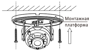
Рисунок 2-3 Установка монтажной платформы
