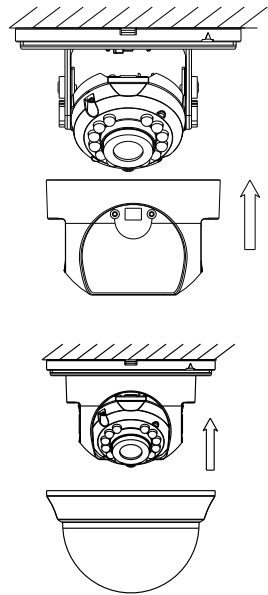
Рисунок 2-5 Завершение установки
