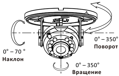
Рисунок 2-4 3-х осевая установка
