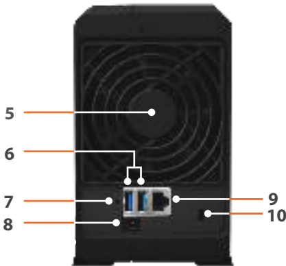
Задняя панель
