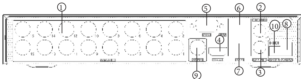
Задняя панель CTV-HD9216 HP Lite
