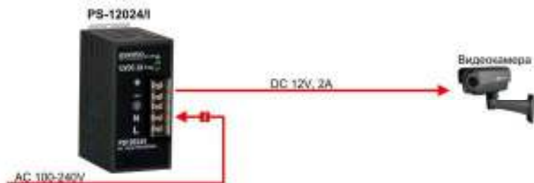
Рис. 4 Подключение PS-12024/I
