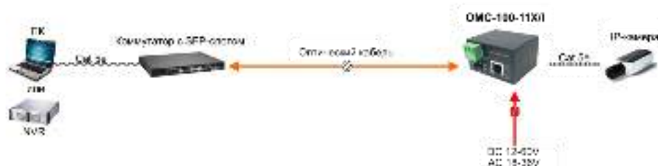
Рис. 6 Схема подключения ОМС-100-11Х/І
