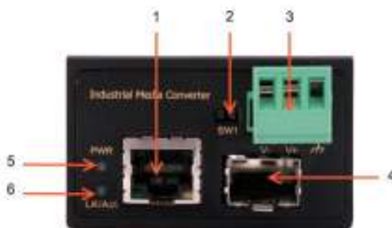
Рис. 2 Разъемы и индикаторы панели подключения ОМС-100-11Х/І
