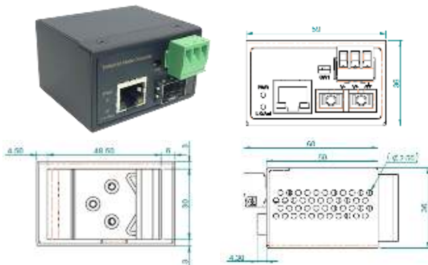
Рис. 1 Внешний вид и габариты ОМС-100-11Х/І
