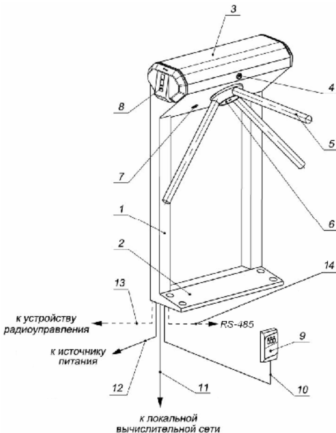
Рисунок 1 Устройство ЭП:
