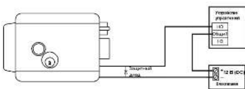
Рис. 10 Схема подключения
