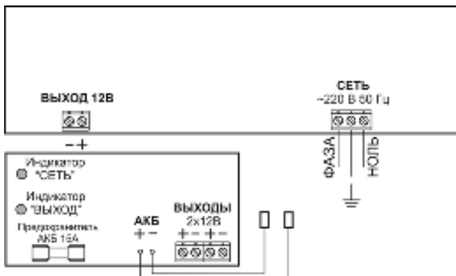
Рисунок 1 — схема подключения изделия
