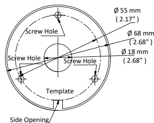
Рис. 2-1 Шаблон крепления
