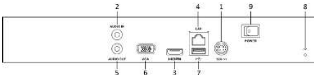
Рисунок 1.3 Задняя панель
