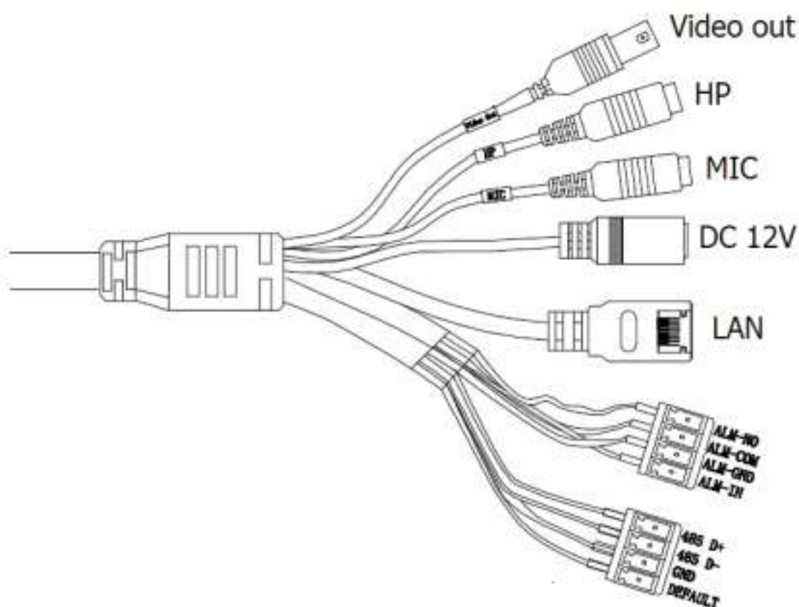
Рис.2.1. Разъемы LTV-ICDMx-E6231L-V
